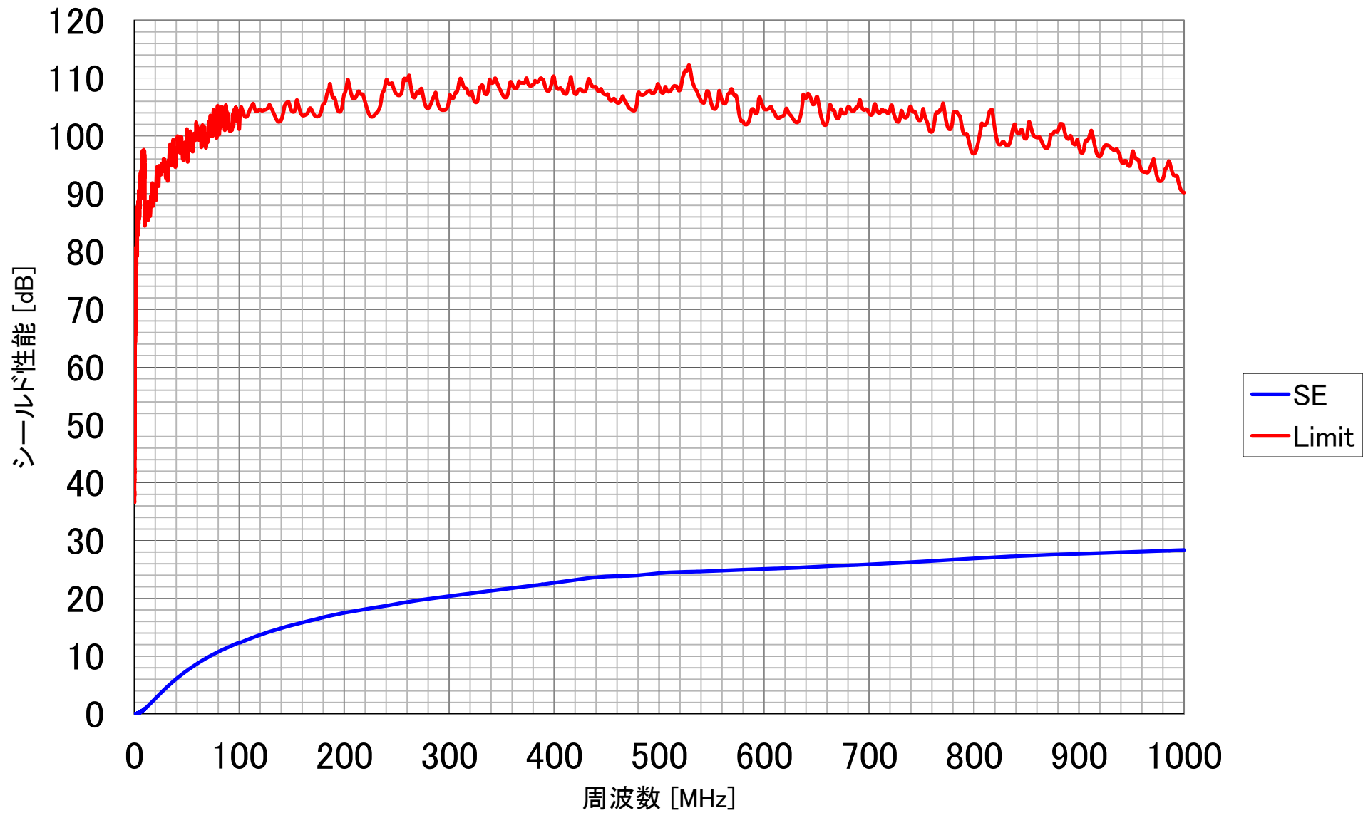
20150303[PCS-107AgCu(40 \mu m)]KEC 法 磁界
