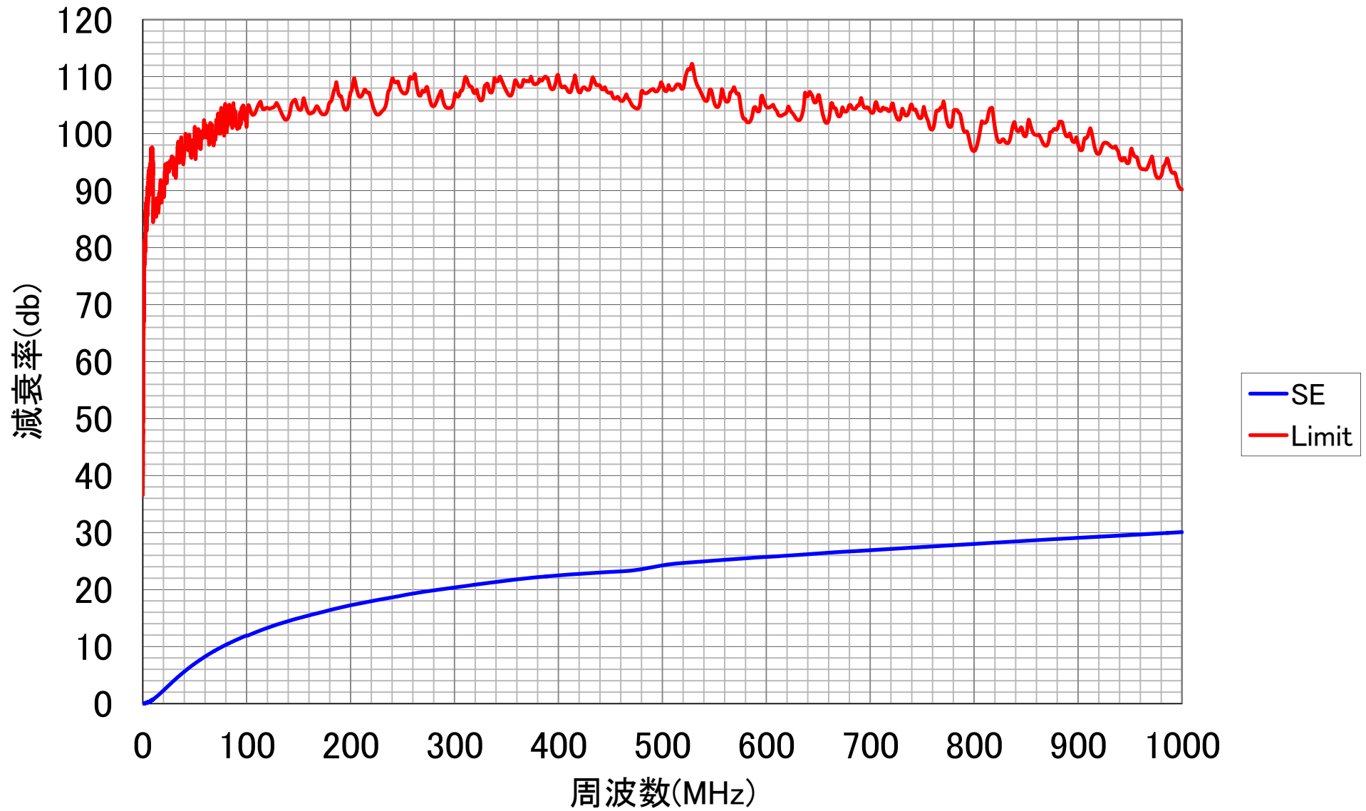
20150303[Polycalm-G1501(35 \mu m)] KEC法 磁界
