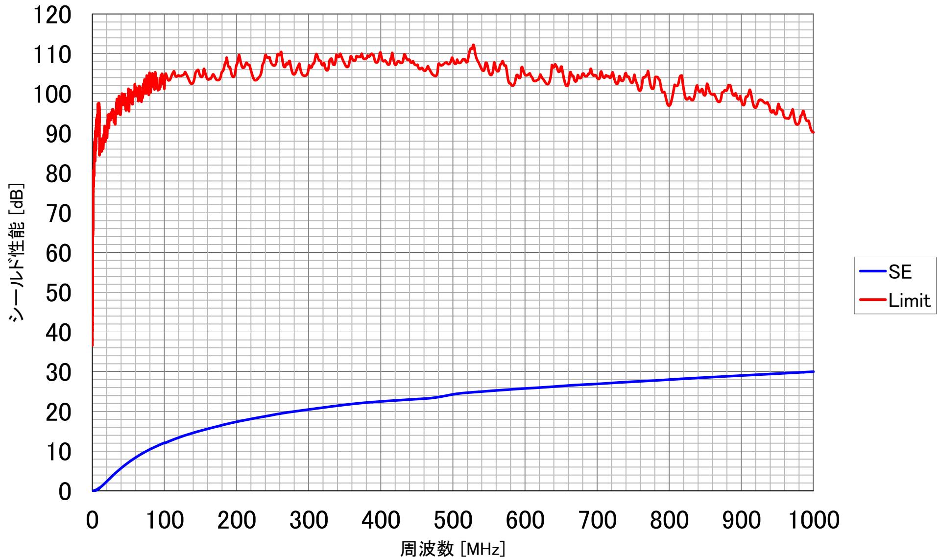
20150303[PCS-104n Ni(45 \mu m)]KEC 法 磁界
