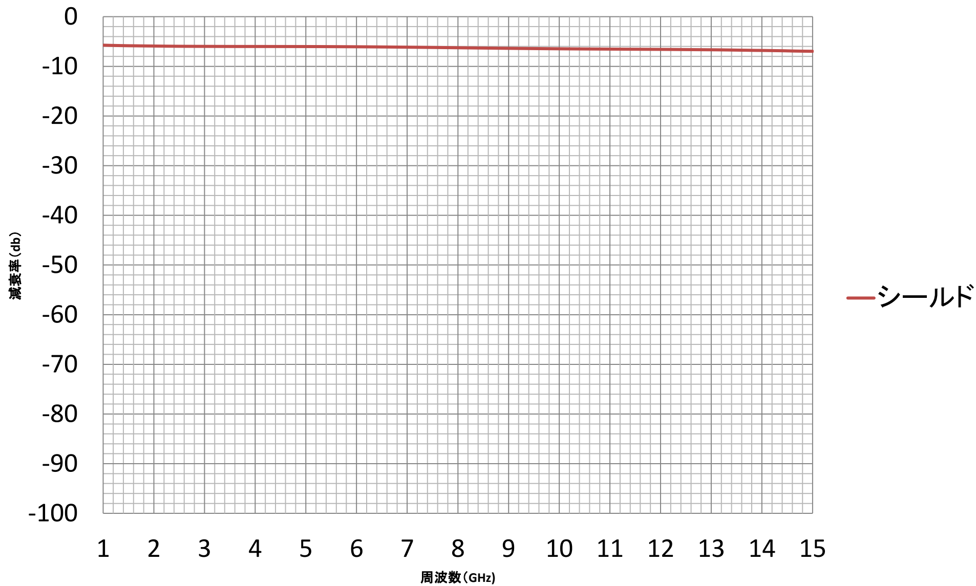
20210908-06_DFFC_1-15GHz_PCS-1949CG_55μ
